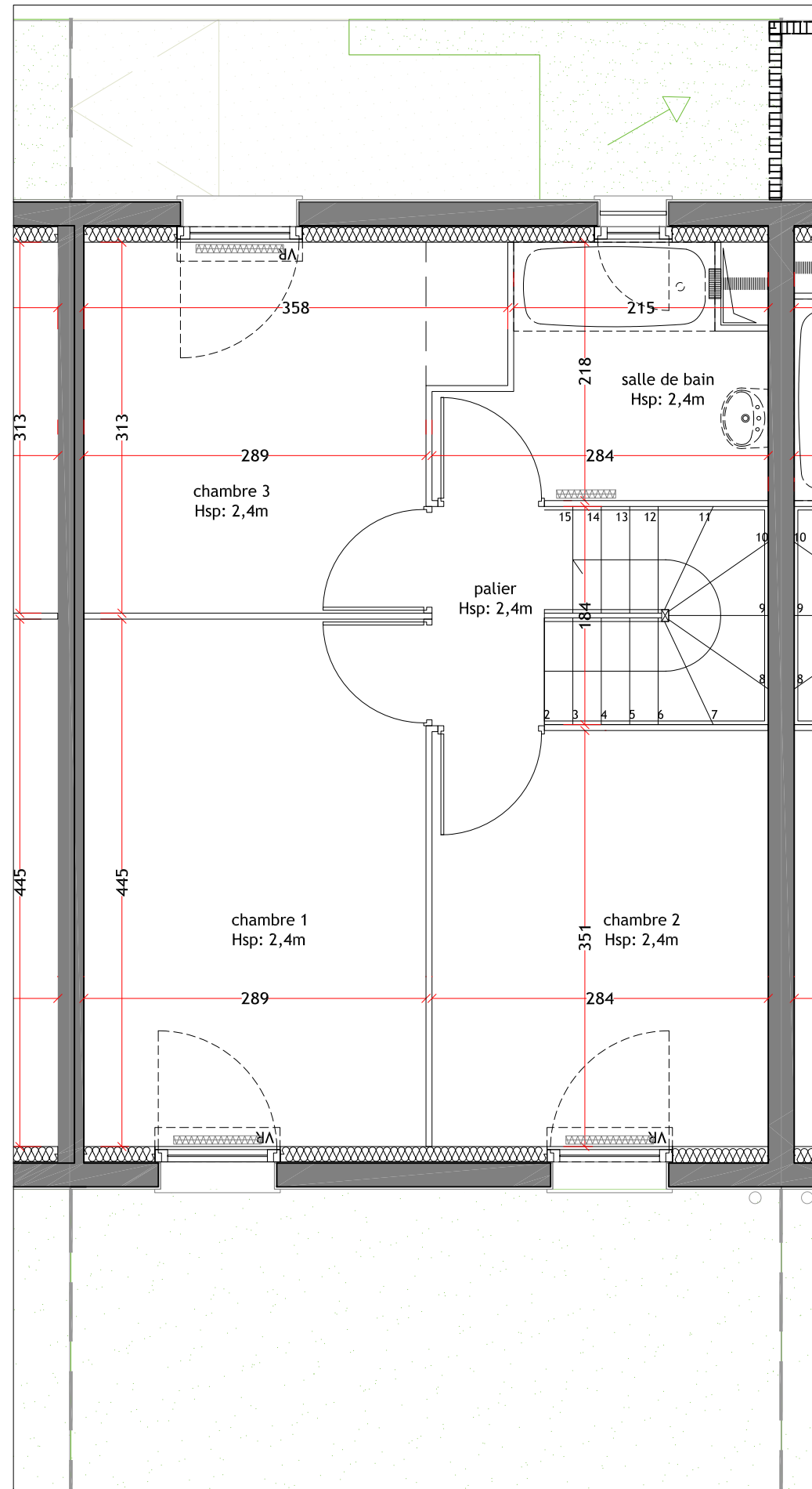
Niveau R+1
