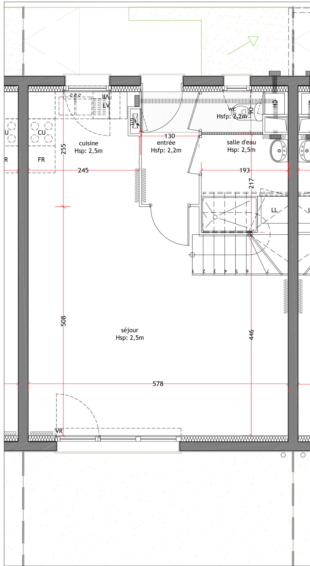
Niveau Rez-de-chaussée
